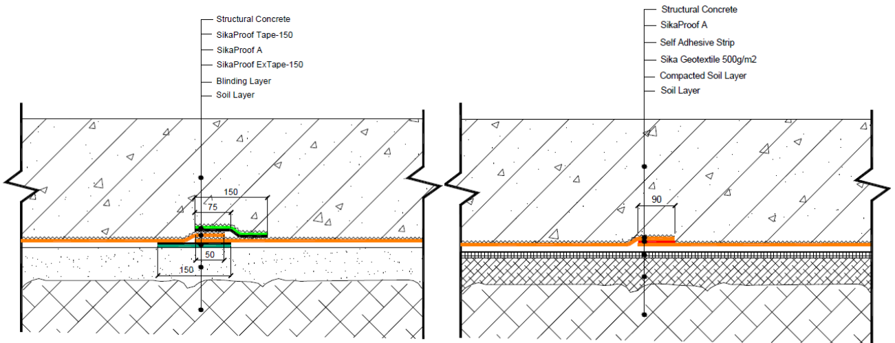
Şekil 2: SikaProof membran temel uygulama detayları
