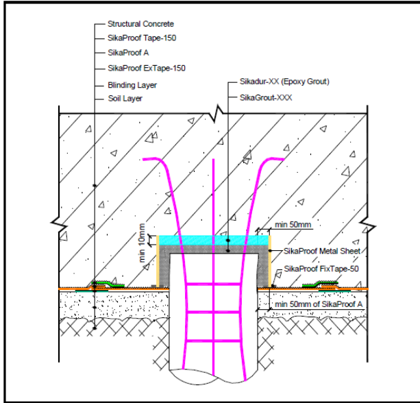
Şekil 6: SikaProof A membran, kazık başı detayları
