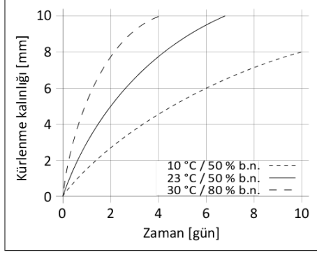
Şekil 1: Sikaflex®-255 FC için kürlenme hızı
